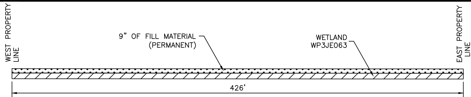
CROSS SECTION #1 N.T.S.
