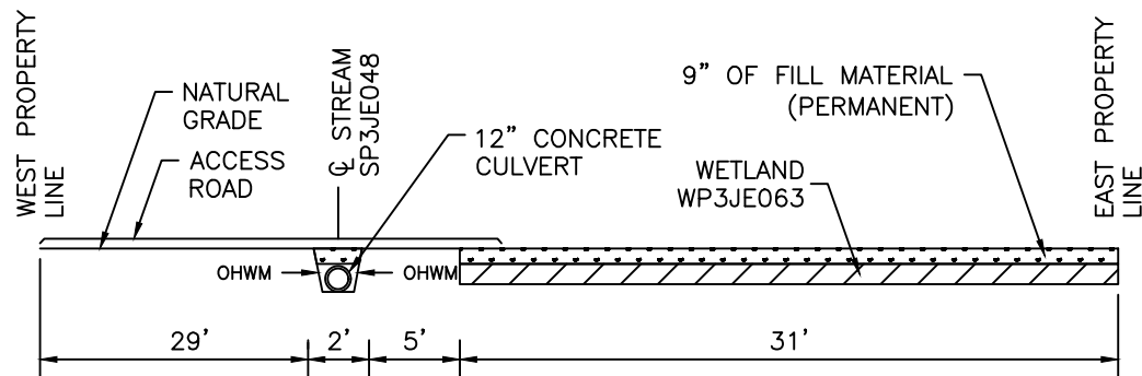
CROSS SECTION #3 N.T.S.
