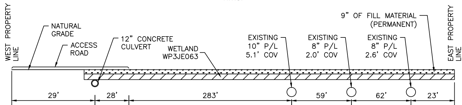
CROSS SECTION #2 N.T.S.
